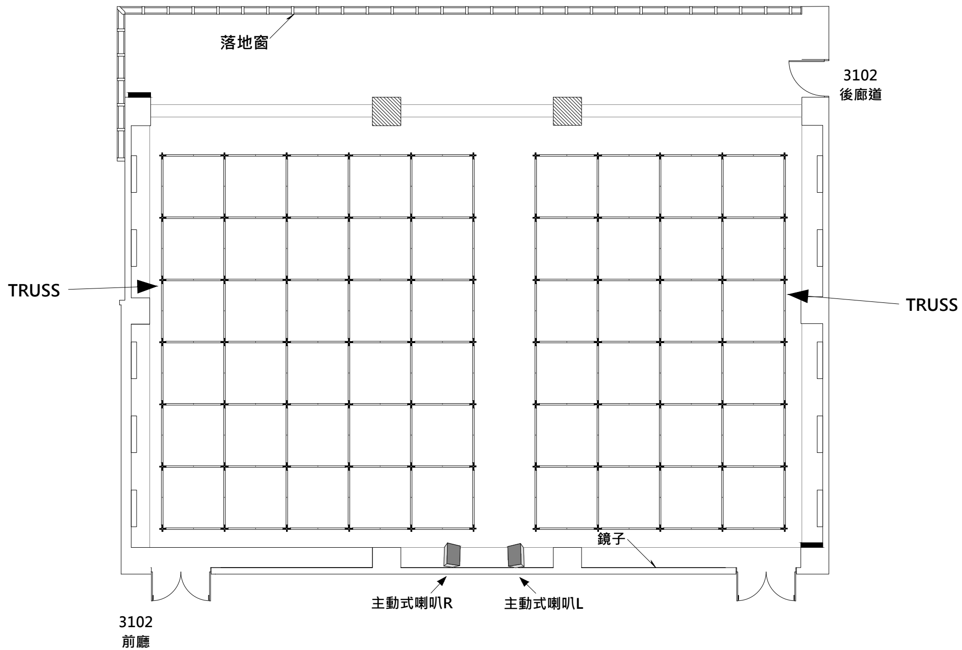
圖 (七) 多功能廳_音響配置圖 (單位: 公分) Figure(7) Multi Hall _ Audio Plan (Unit: cm)
